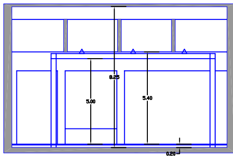
Sección transversal
